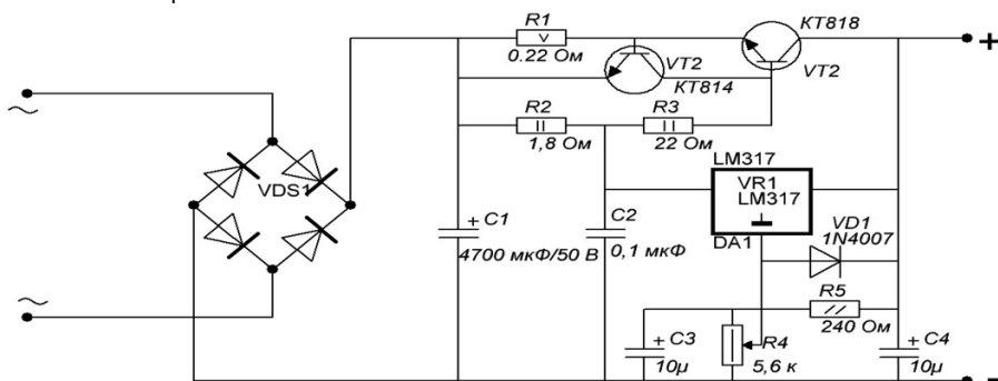
Рисунок 1 – Принципиальная схема регулируемого источника питания
