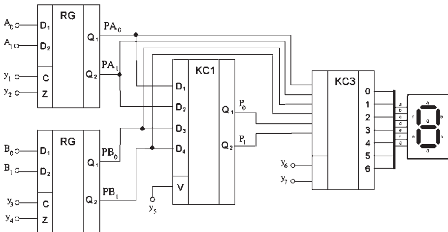
Рис. 1. Функциональная схема проектируемого АЛУ
