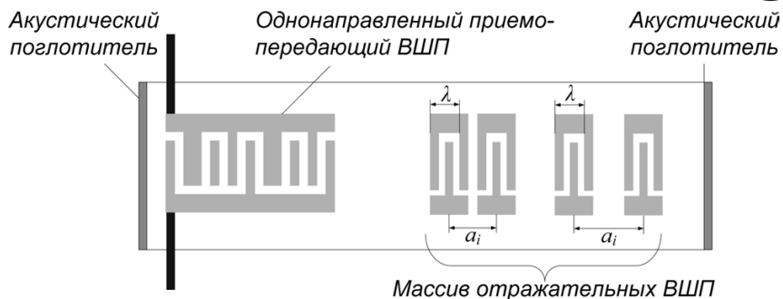
Рисунок 1 – Конструкция радиочастотной идентификационной метки на ПАВ
