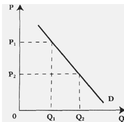
Рисунок 1. Кривая спроса
